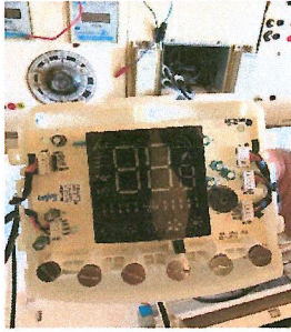
Hantech Salon Tipi Klima İç Ünite Kartı resmi
