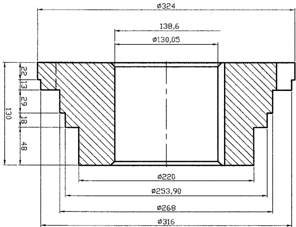
A-A KESİTİ
